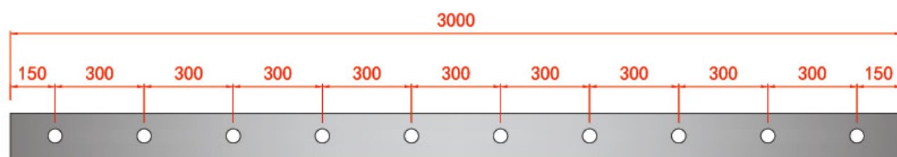
内侧 INSIDE 俯视图 TOP VIEW
