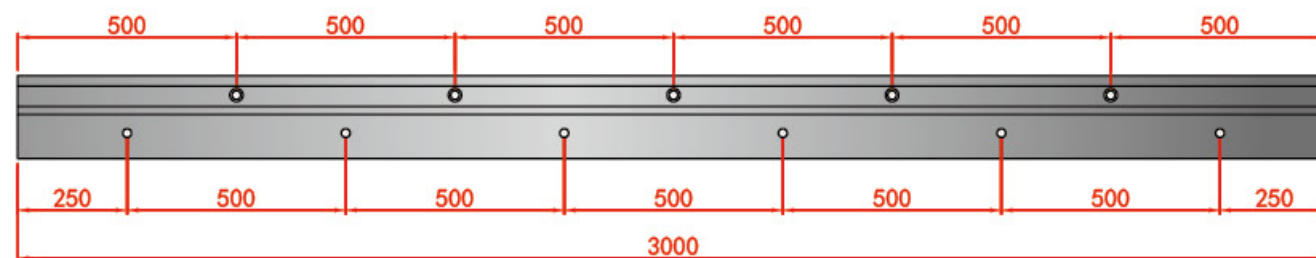
内側 INSIDE 俯视图 TOP VIEW
