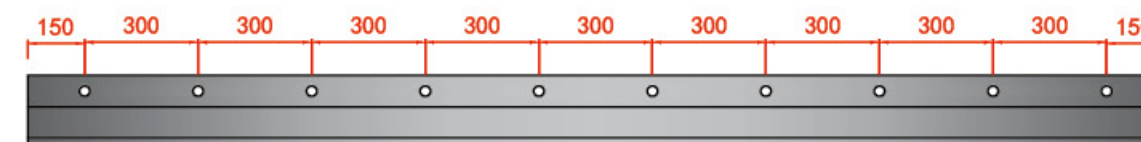
外侧 俯视图 OUTSIDE TOP VIEW
