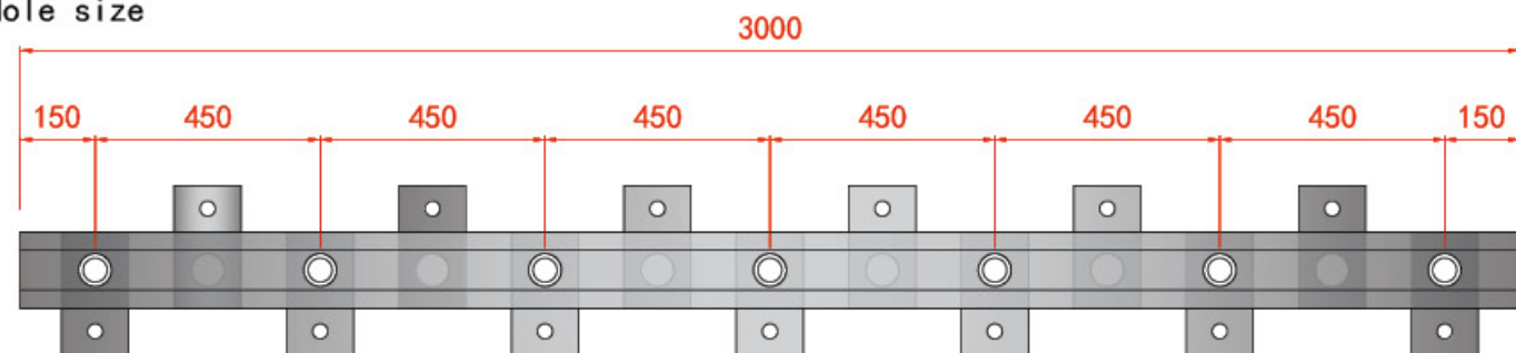
内侧 俯视图 INSIDE TOP VIEW
