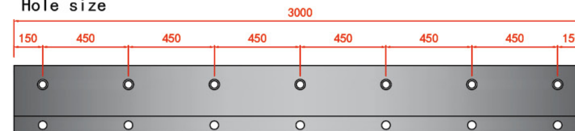
正视图 FRONT VIEW
