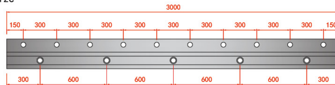
正视图 FRONT VIEW
