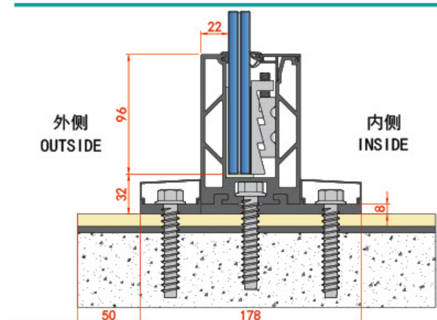
开孔尺寸 Hole size
