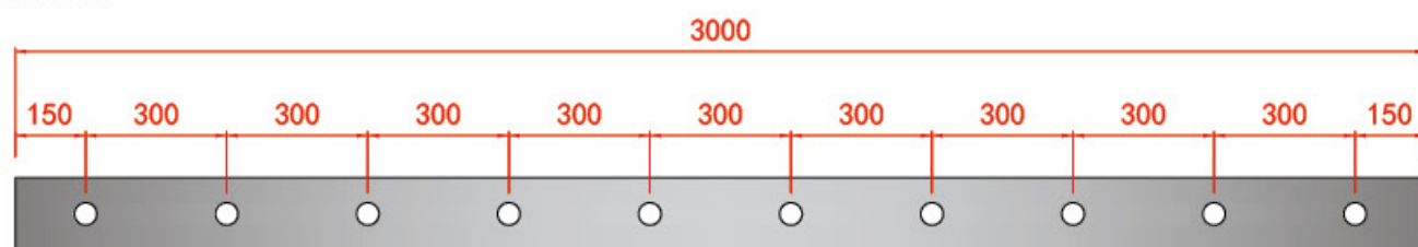
开孔尺寸 Hole size
