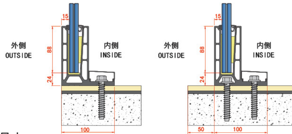
开孔尺寸 Hole size
