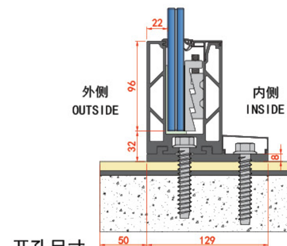
开孔尺寸 Hole size
