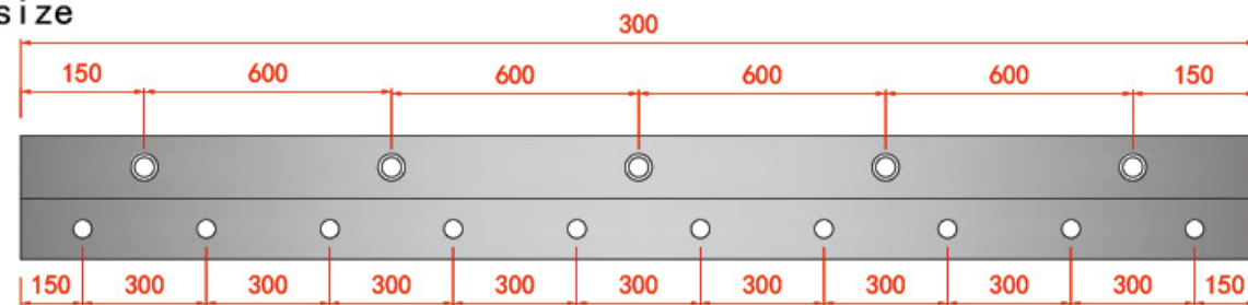
內側 INSIDE 俯视图 TOP VIEW
