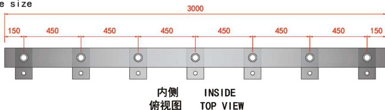
开孔尺寸 Hole size
