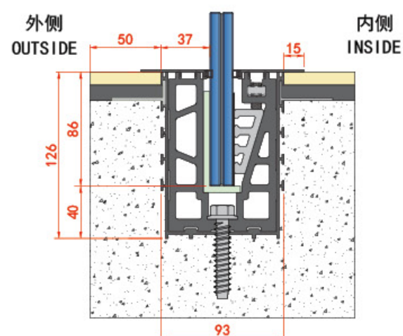
开孔尺寸 Hole size
