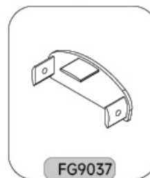
FG9037 扶手管端盖 End Cap
