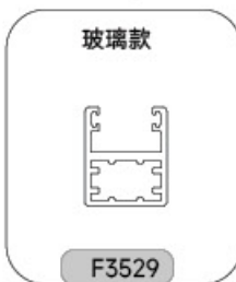
F3529 底部型材 Bottom profile
